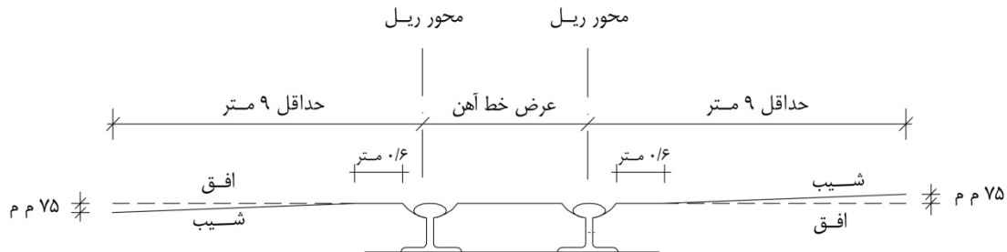
شکل ۸-۵۰- تقاطع راه- راه‌آهن
