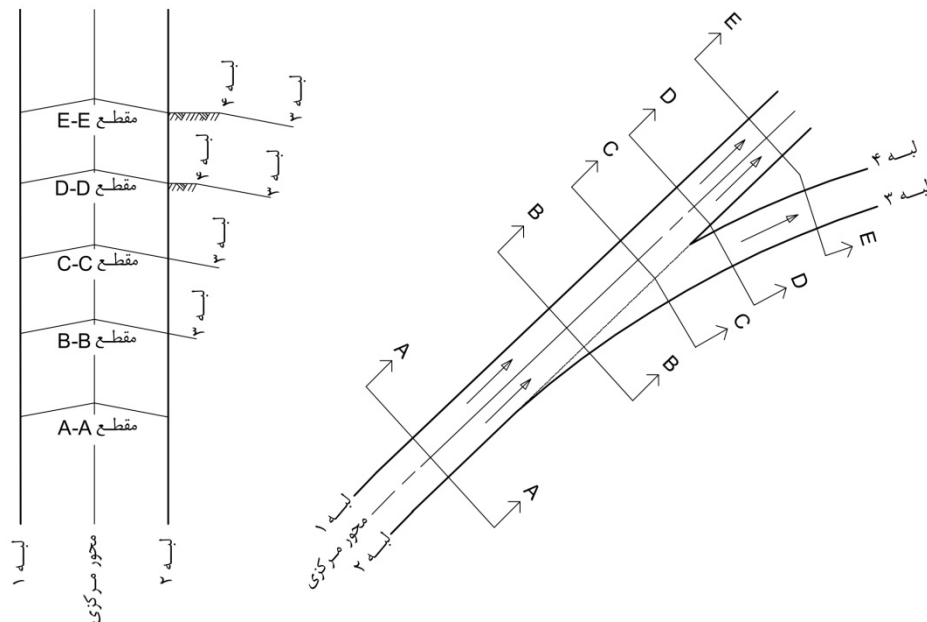
شکل ۸-۲۹- نحوه تأمین برابندی در پایانه- جدانشدگی از خط مستقیم
