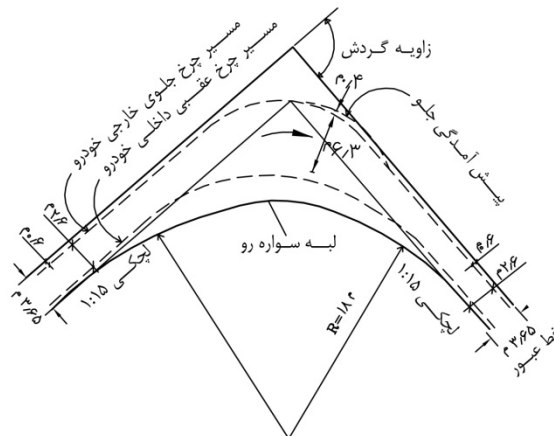
حداقل طرح با قوس ساده و لیجکی به شعاع ۱۸ متر با عقب نشینی ۱ متر
